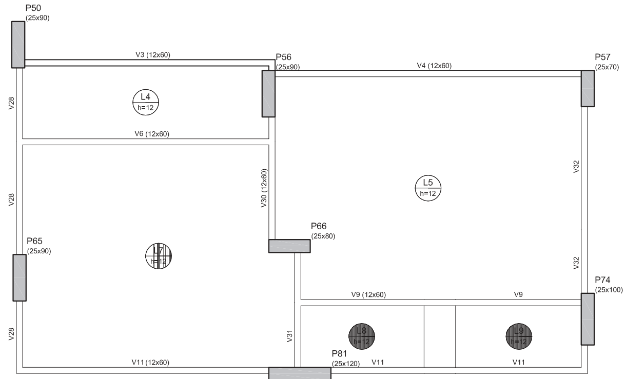
PLANTA DE FORMA- ESTRUTURA
