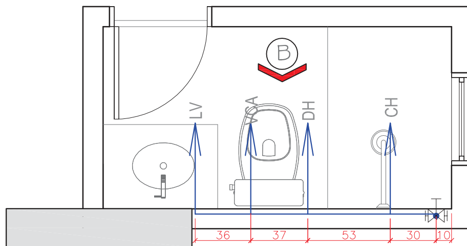
PLANTA BAIXA B.SOCIAL - ÁGUA
