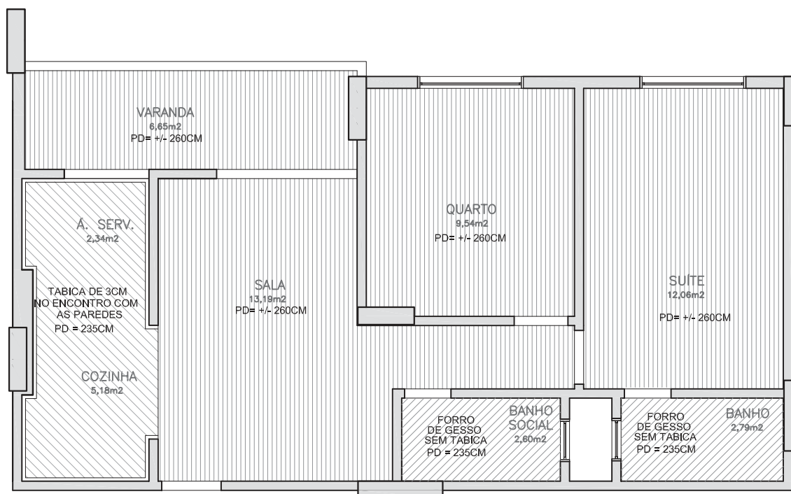
PLANTA DE GESSO 0 1 2 3 4m Escala Gráfica em metros
