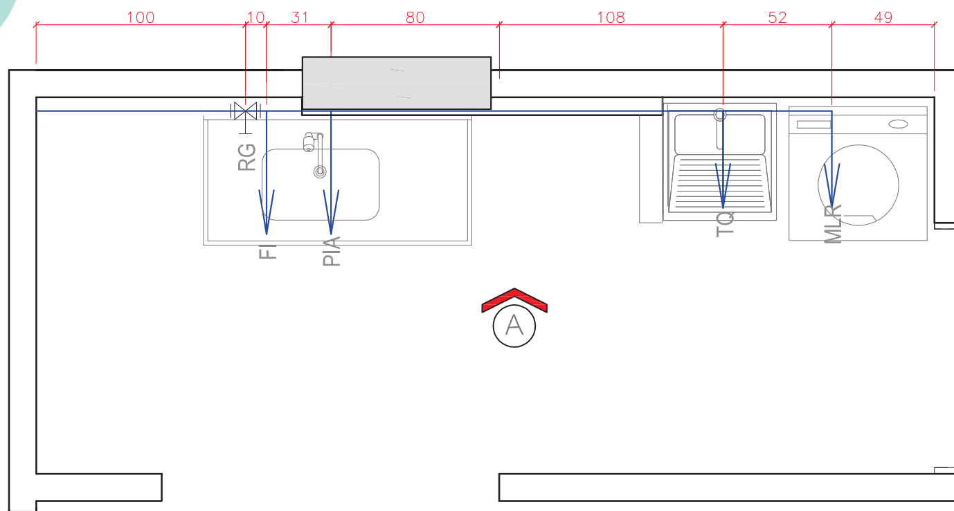
PLANTA BAIXA COZINHA - ÁGUA
