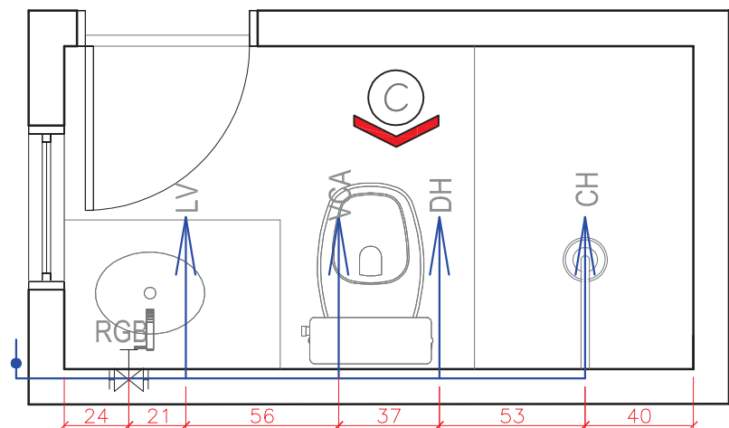
PLANTA BAIXA B.SUÍTE - ÁGUA
