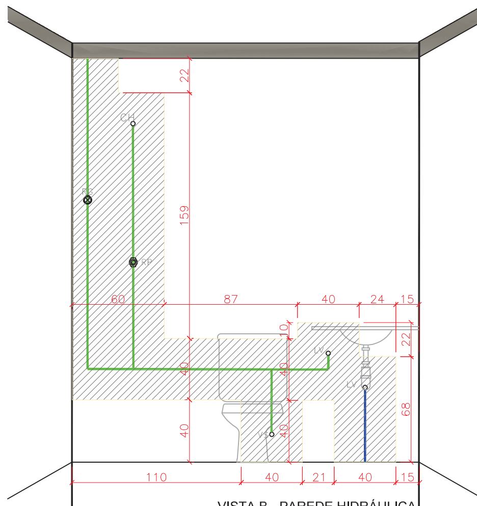
VISTA B - PAREDE HIDRÁULICA BANHO SOCIAL
