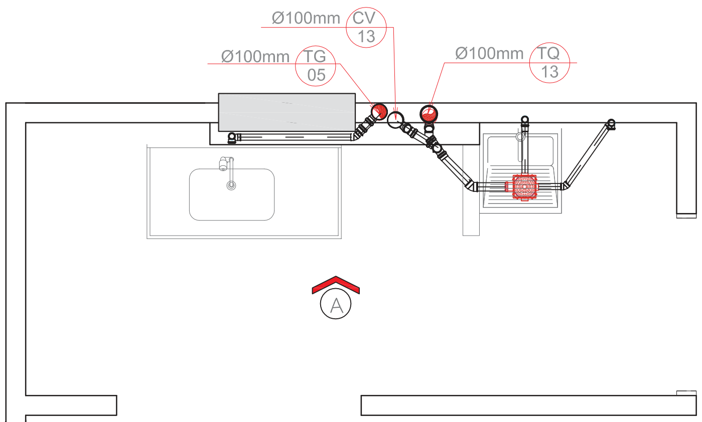
PLANTA BAIXA COZINHA - ESGOTO
