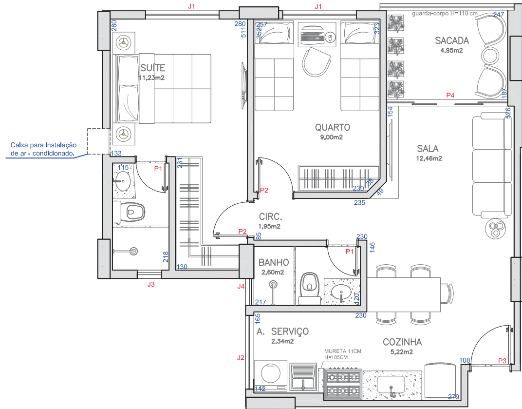
PLANTA ALVENARIA
