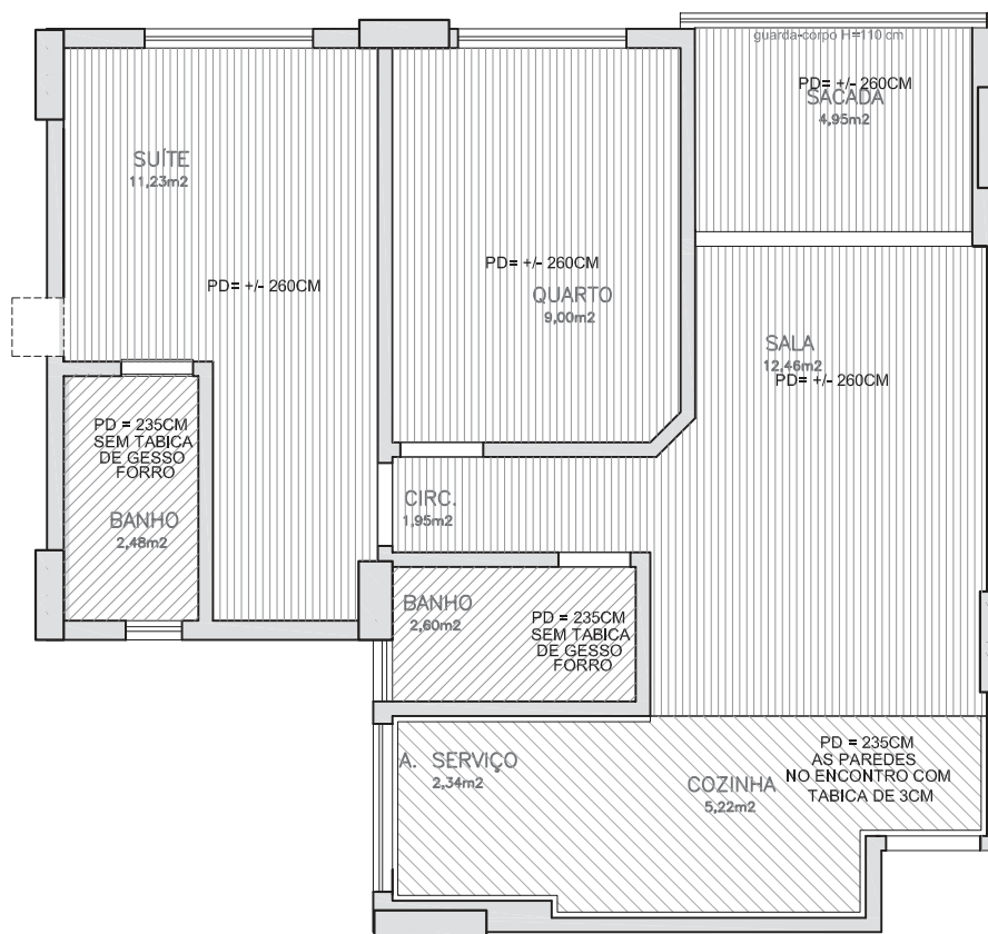
PLANTA DE GESSO
