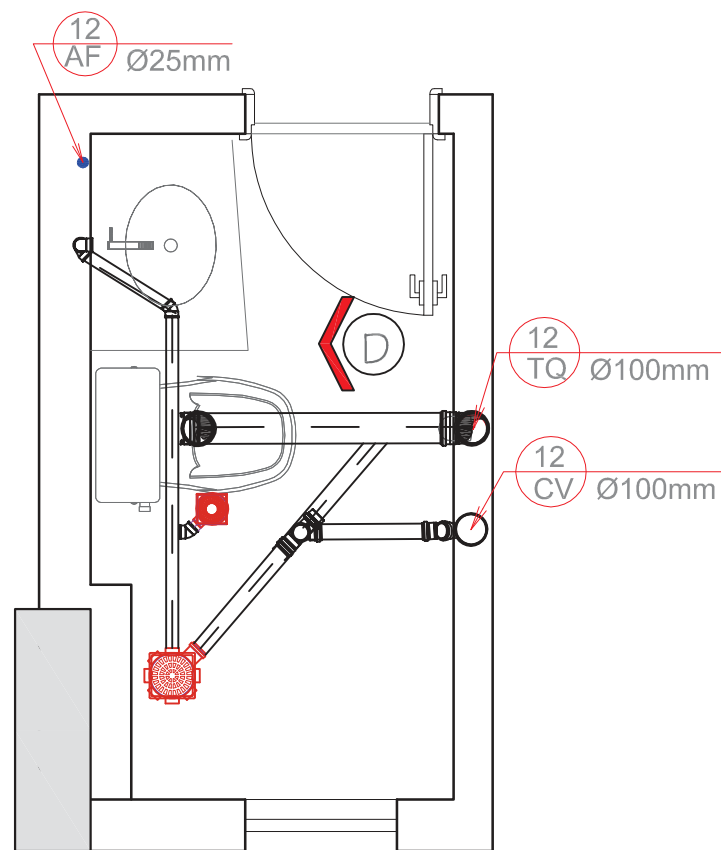
PLANTA BAIXA B.SUÍTE - ESGOTO
