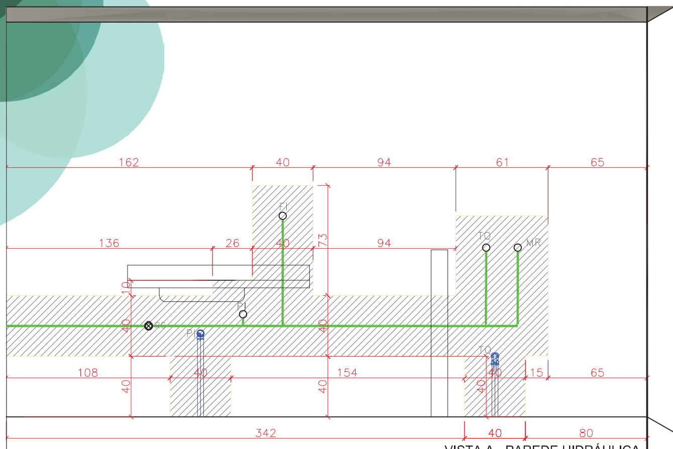
VISTA A - PAREDE HIDRÁULICA COZINHA
