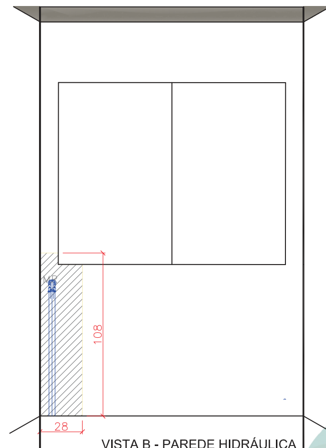
VISTA B - PAREDE HIDRÁULICA COZINHA
