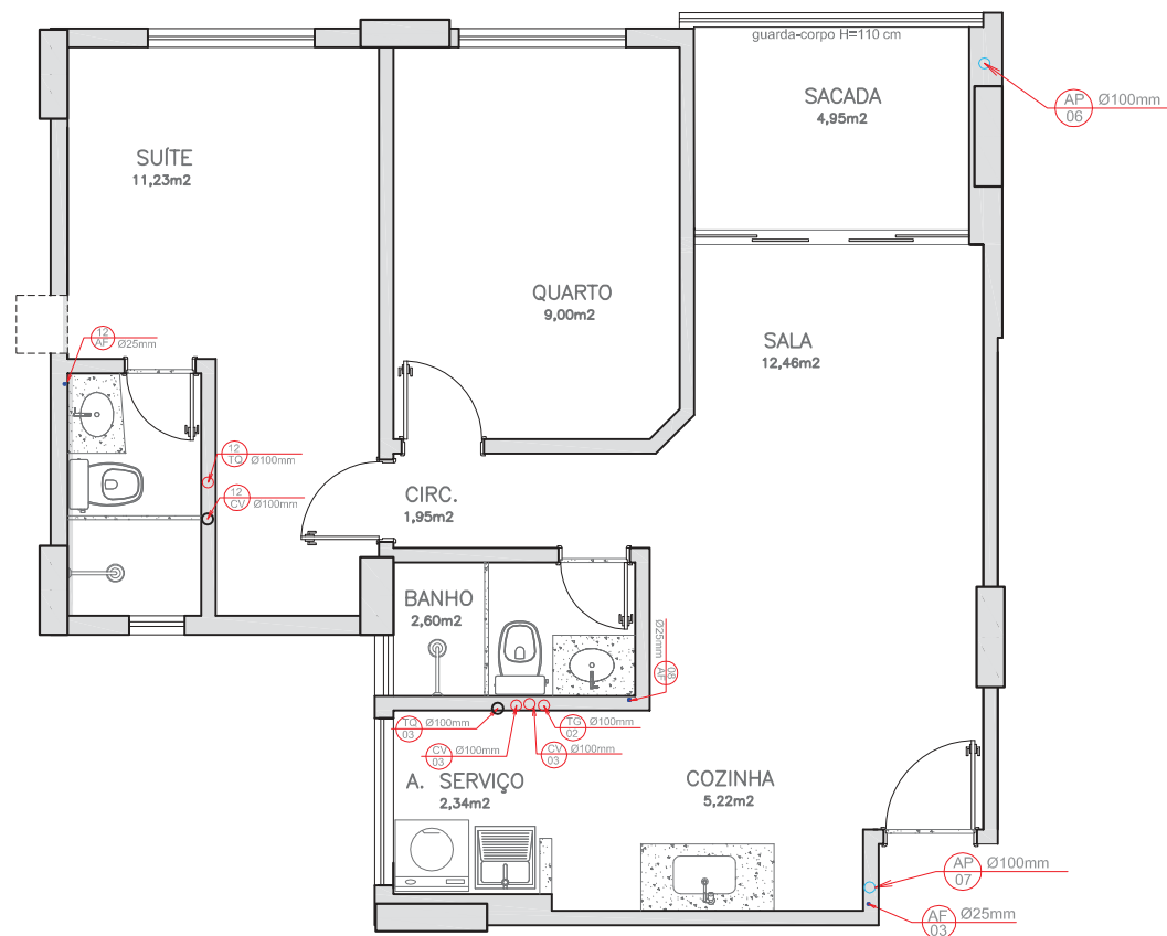
PLANTA HIDRO-SANITÁRIA
