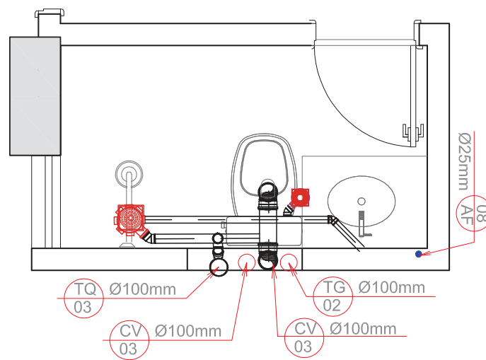
PLANTA BAIXA B.SOCIAL - ESGOTO
