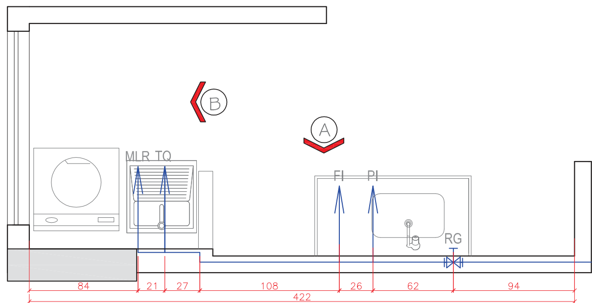
PLANTA BAIXA COZINHA - ÁGUA
