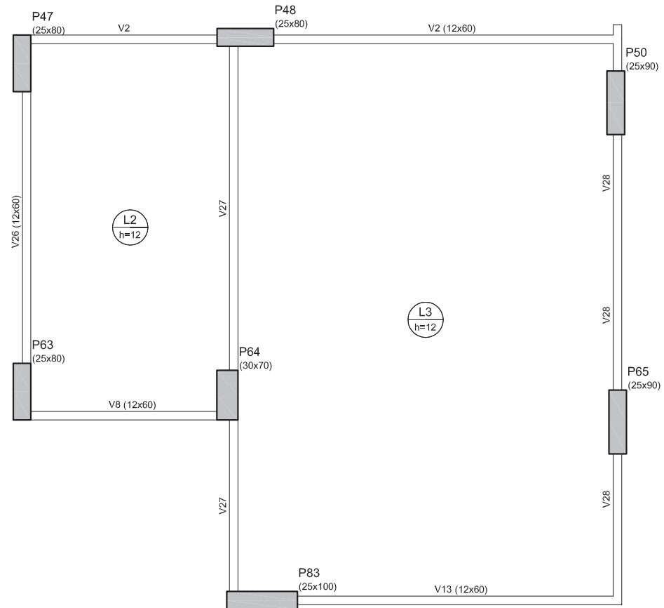
PLANTA DE FORMA- ESTRUTURA
