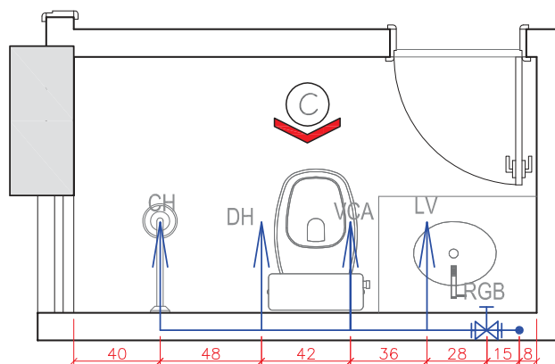
PLANTA BAIXA B.SOCIAL - ÁGUA
