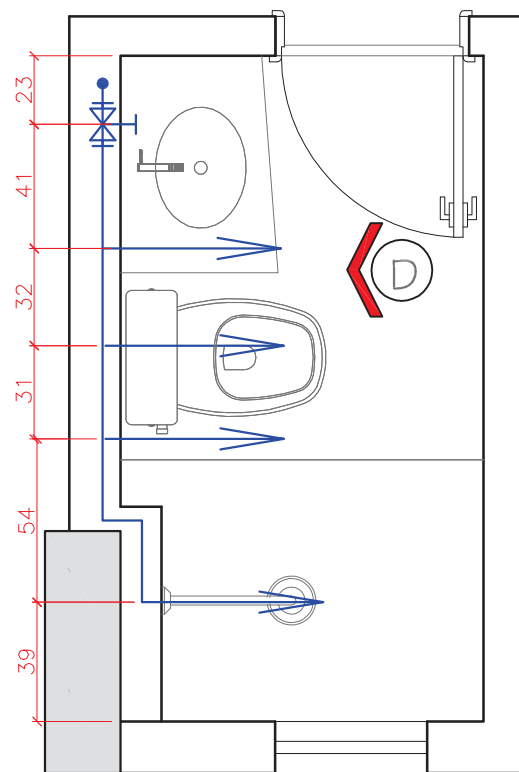
PLANTA BAIXA B.SUÍTE - ÁGUA
