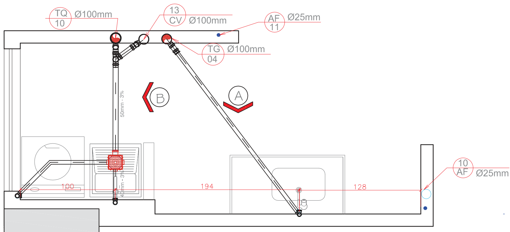
PLANTA BAIXA COZINHA - ESGOTO
