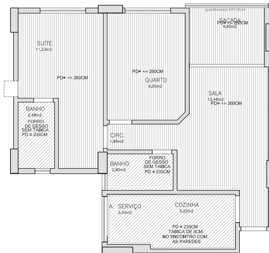
PLANTA DE GESSO
