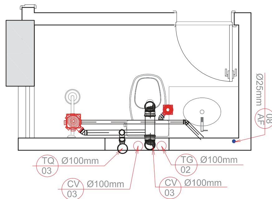
PLANTA BAIXA B.SOCIAL - ESGOTO
