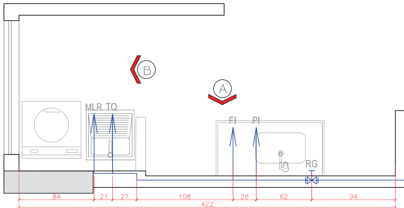
PLANTA BAIXA COZINHA - ÁGUA
