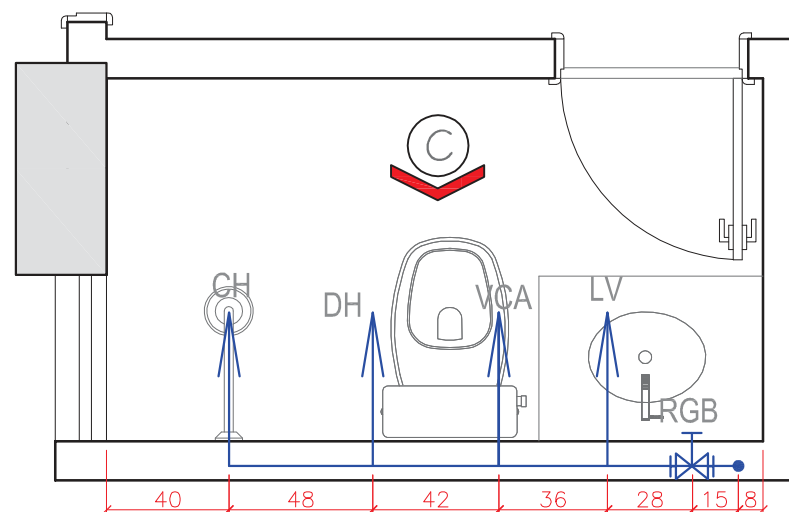
PLANTA BAIXA B.SOCIAL - ÁGUA
