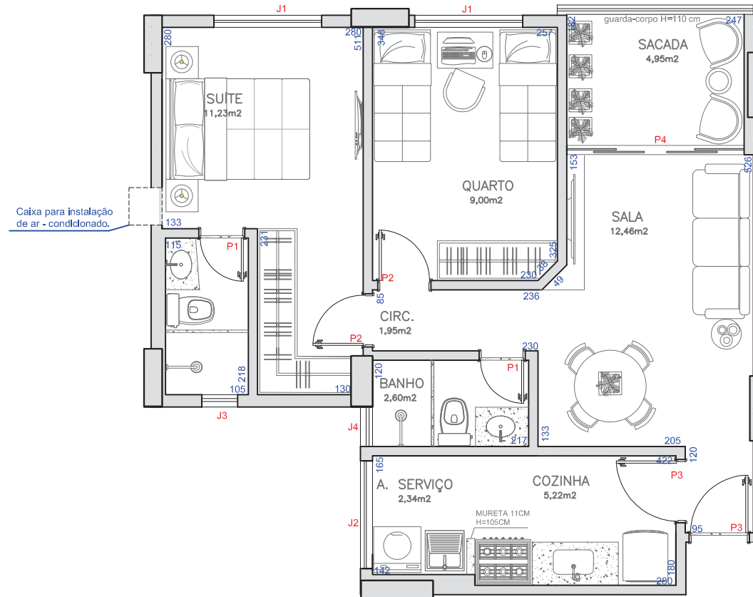
PLANTA ALVENARIA
